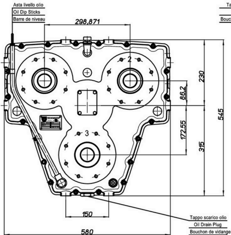
TMP 341 Dimensioni
