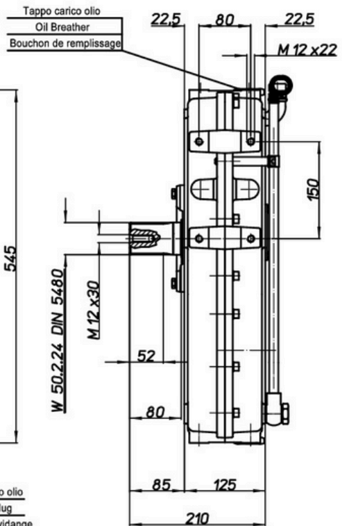
TMP 341 Dimensions
