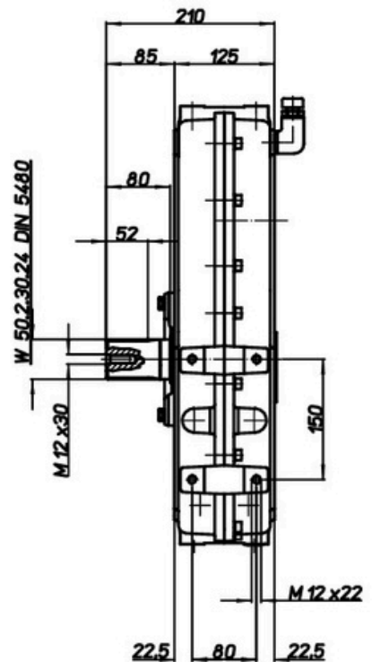
TMP 340 Dimensions
